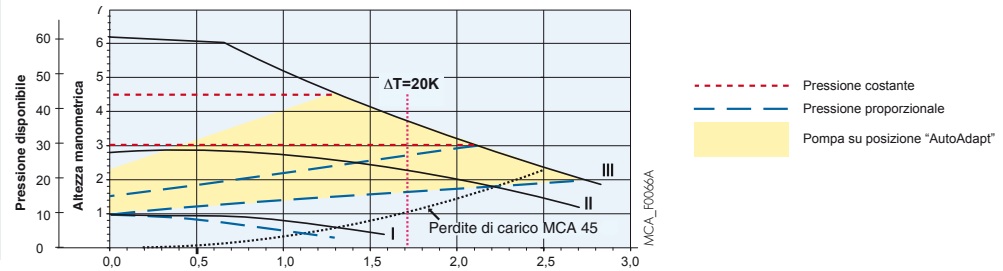
Pompa primario per MCA 45 e 65 - Collo HC 147 (consegnata con 2 raccordi di collegamento) Questa pompa può anche fungere da pompa primaria negli impianti in cascata. Caratteristiche della pompa UPS 25-55 180
