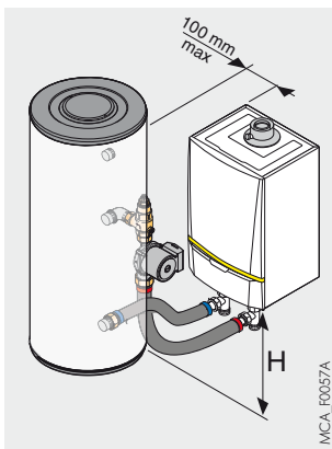
Kit di collegamento caldaia MCA 45, 65, 90 e 115 /bollitori BP/BL..., UNO/2, DUO/2 o TRIO - Collo EA 121
