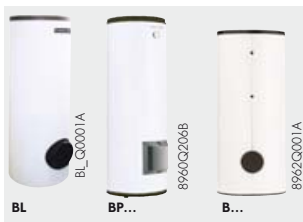
Produzione dell'acqua calda sanitaria I bollitori indipendenti De Dietrich della serie B..., con capacità da 150 a 1000 litri, consentono di produrre acqua calda sanitaria per abitazioni singole e collettive ed anche per locali industriali e commerciali. Sono protetti al loro interno da smalto vetrificato ad alto contenuto di quarzo, per
