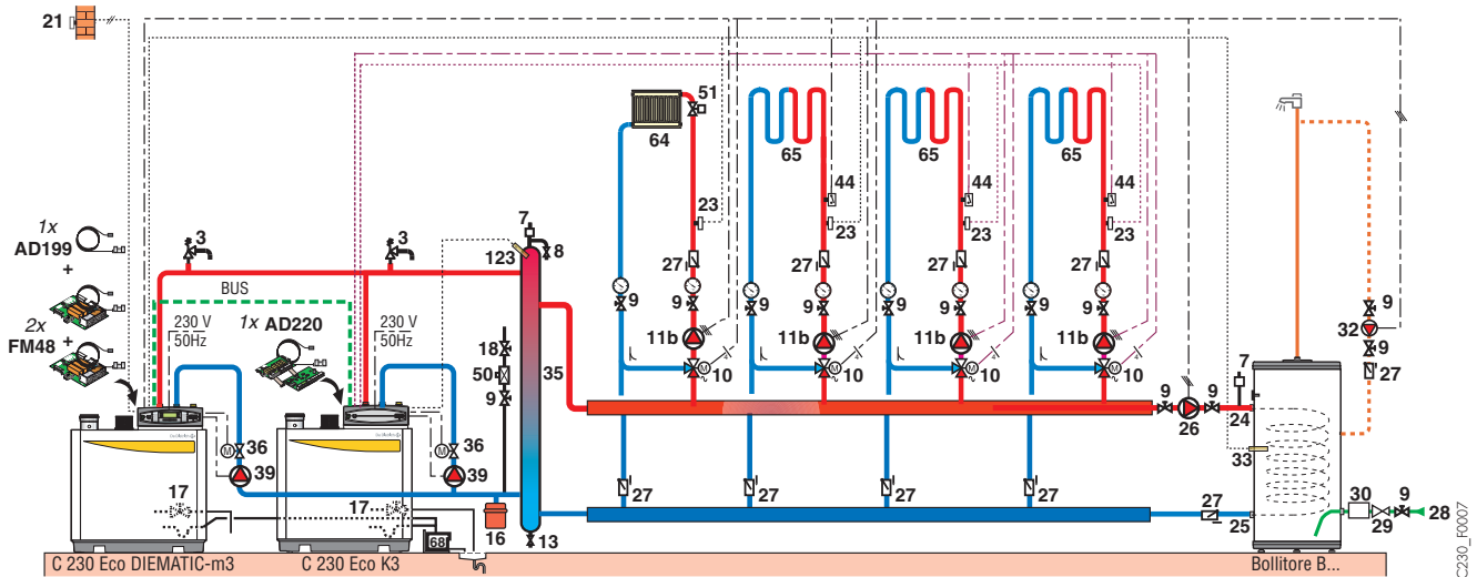
Installazione di 2 caldaie in cascata (circuito primario di tipo 1 con pompe d'iniezione) con 4 circuiti con valvola miscelatrice + 1 circuito di acqua calda sanitaria, tutti dietro un compensatore idraulico
